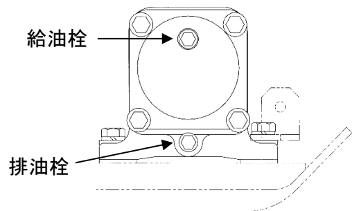
起振体側面
